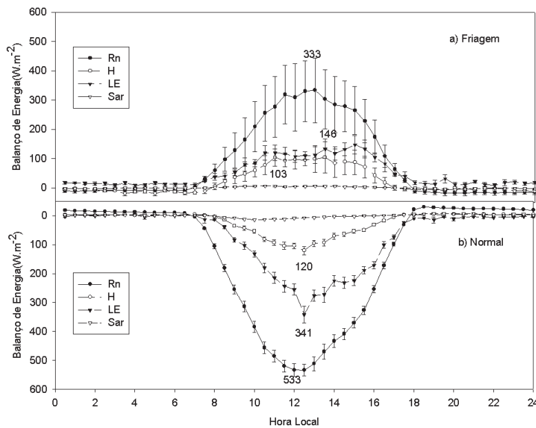
Figura 5 - Ciclo Diurno Médio do Balanço de Energia para dias de Friagem (a) e dias Normais (b)
