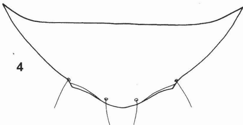
Figures 3-4. Sternite VI of female. Fig. 3. N. viridula . Fig. 4. N. pseudolimbipennis .
