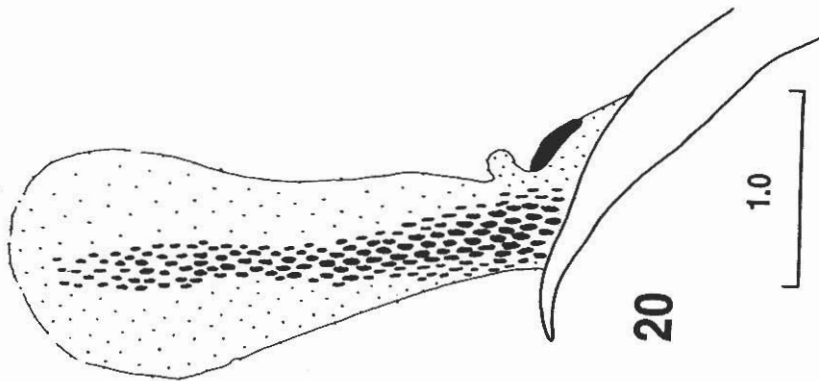
Figures 20-22. Everted internal sac of male genitalia. Fig. 20. N. pseudolimbipennis , Fig. 21. N. maxima , Fig. 22. N. glabrata (scales 1 mm).
